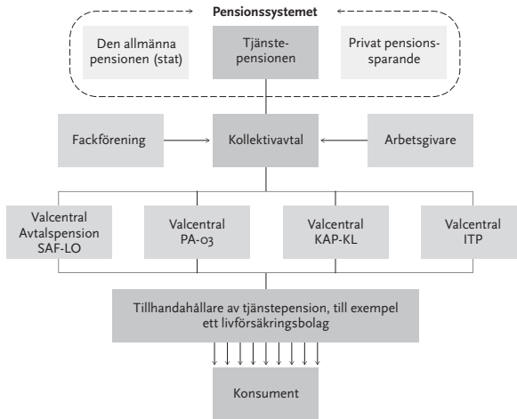
Figur 1. Tjänstepensionssystemet
