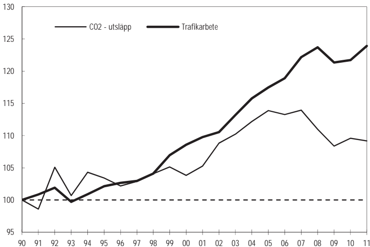
Figur 3.5: Utveckling av trafikarbete på väg och koldioxidutsläpp från vägtrafikerna under åren 1990-2011 relaterat till basåret 1990.
