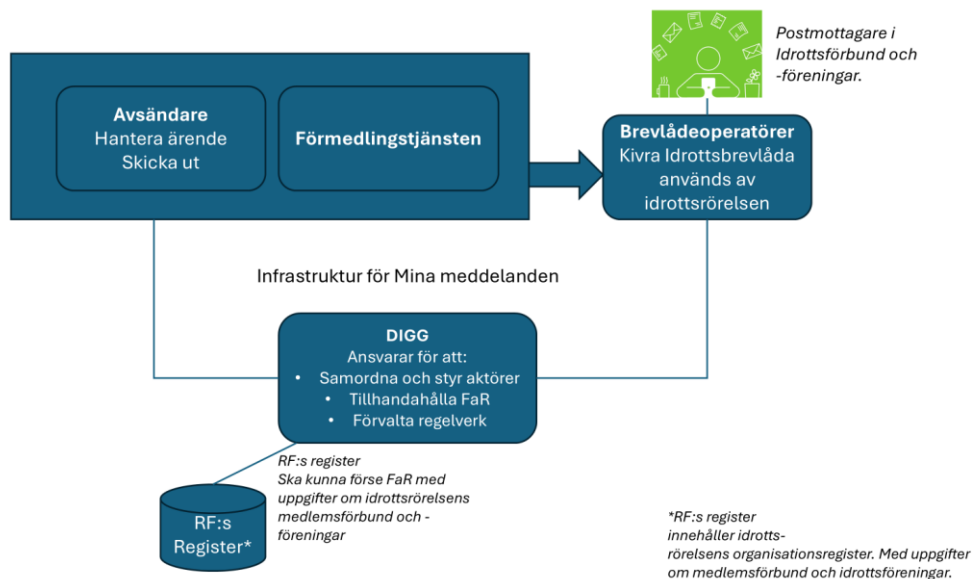
Bild 1. Föreslagen arkitektur för att inkludera idrottsrörelsen i mottagandet av digital post från offentliga aktörer.
