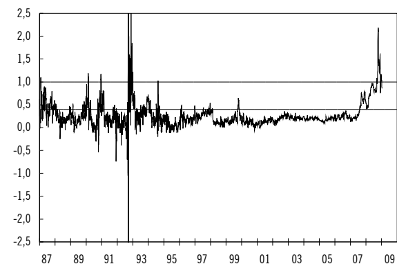
Diagram 3.1 TED-spread Sverige
