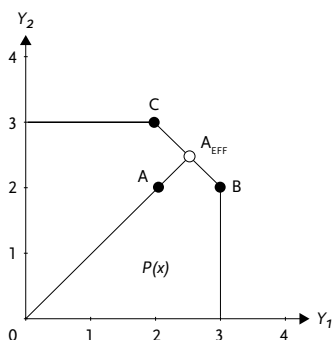
Figur 1. Beskrivning av en outputbaserad DEA-modell
