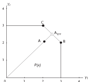
Figur 1 Beskrivning av en outputbaserad DEA-modell
