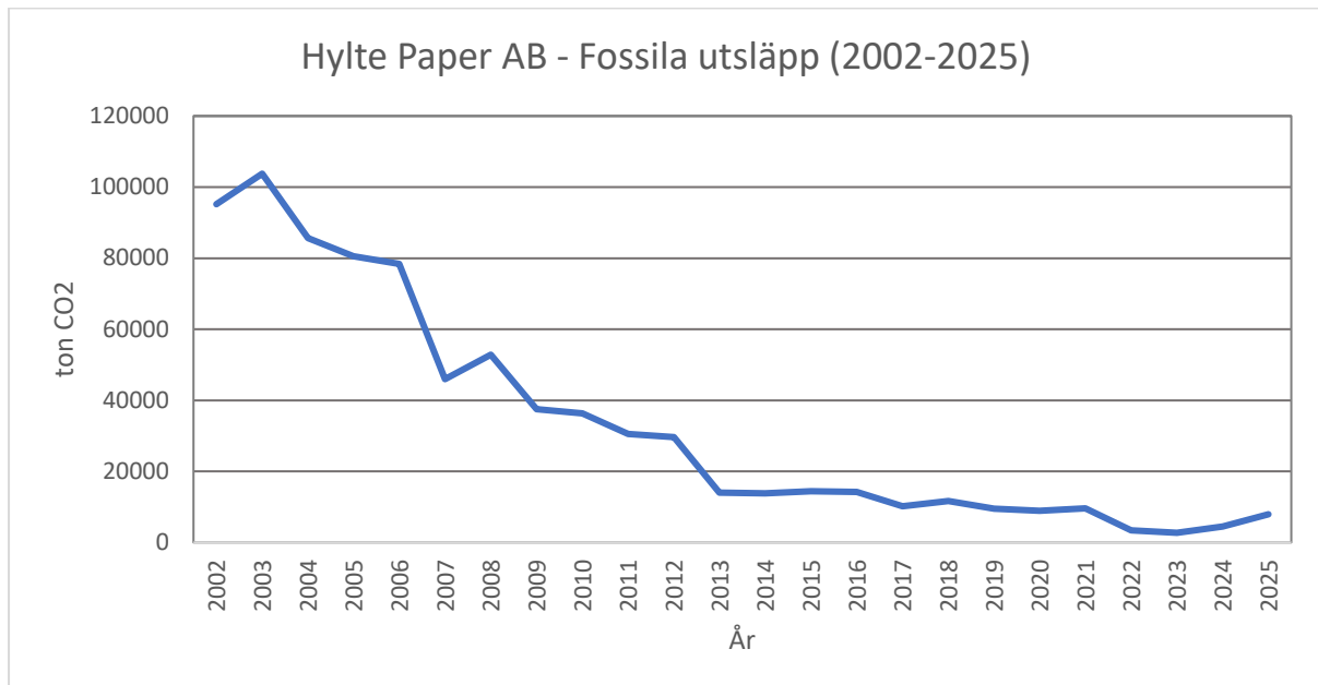
Diagram 1. Fossila utsläpp 2002 – 2025
