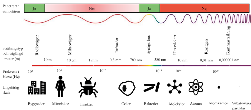
Figur 3.1 Elektromagnetiskt spektrum
